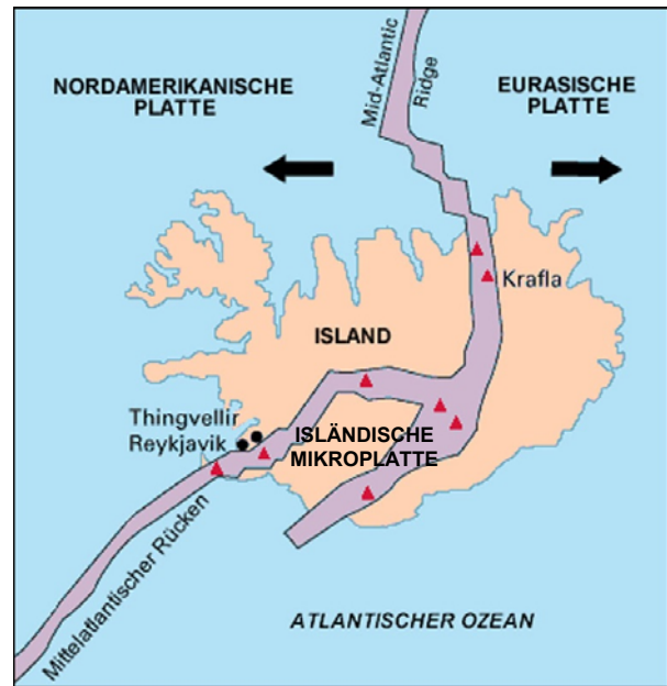
Quer durch Island verläuft der Mittelatlantische Rücken, die platten-tektonische Grenze zwischen Amerika und Europa (?) ... wobei Island sich auf einem gigantischen Manteldiapir befindet
